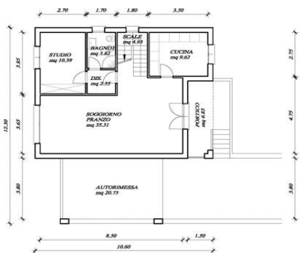
PIANTA PIANO TERRENO
