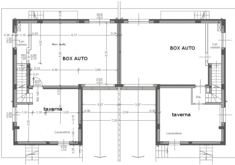
PIANTA PIANO INTERRATO PROGETTO
