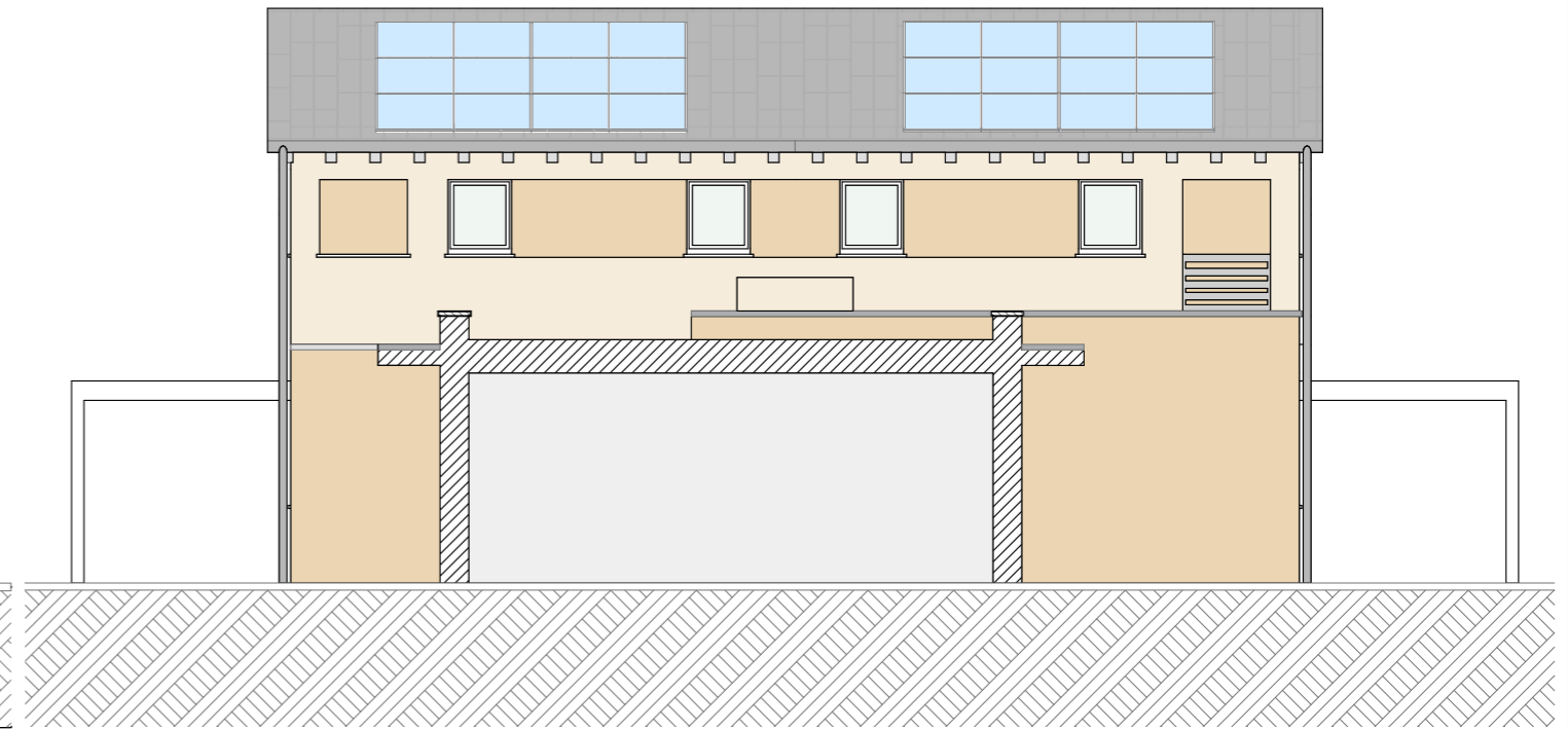
PROSPETTO EST
