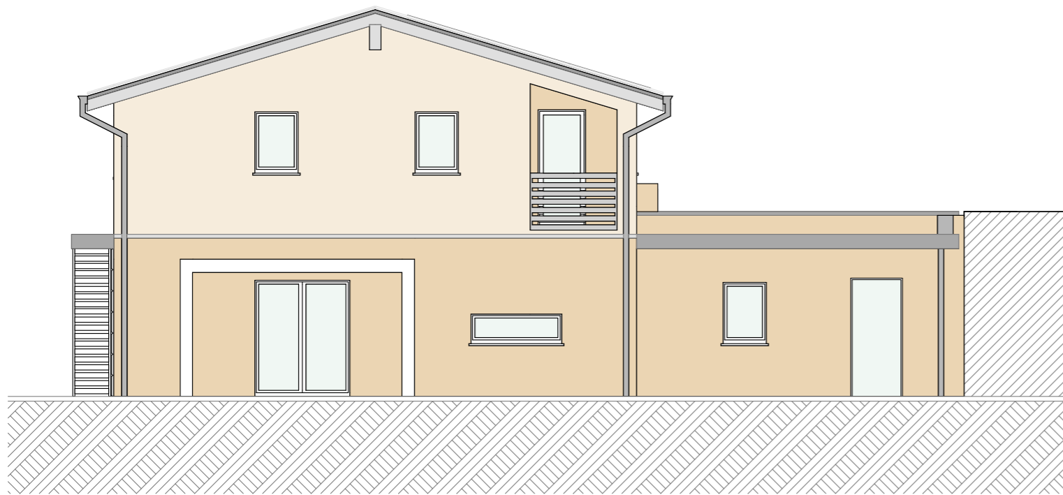
PROSPETTO SUD
